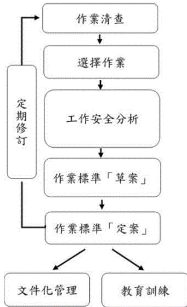
圖一 安全作業標準製作步驟
